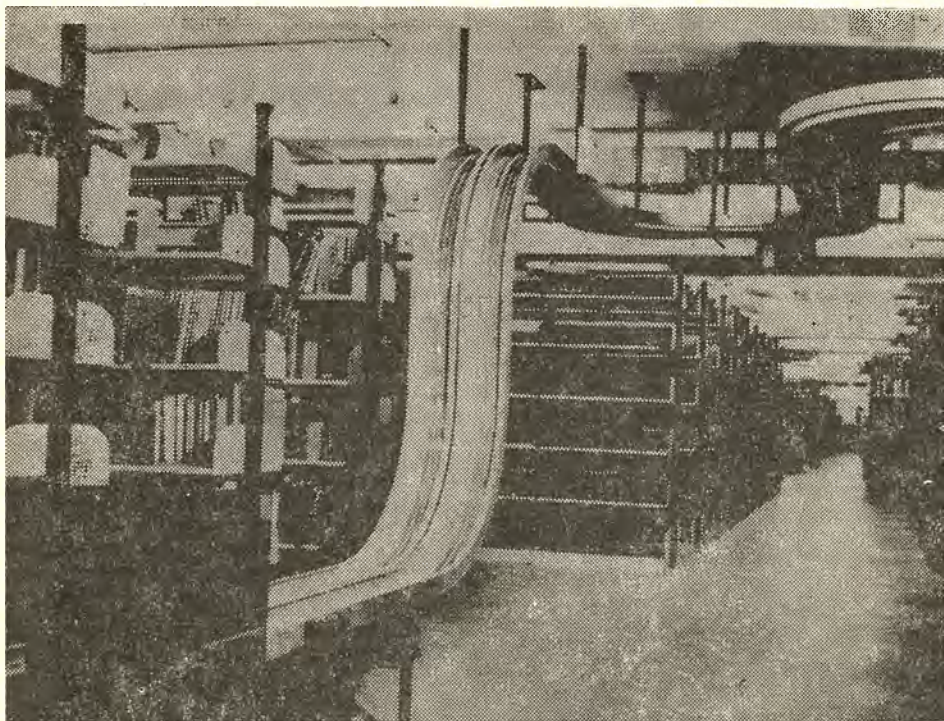
Biblioteka Główna Uniwersytetu w Düsseldorfie. Urządzenia do transportu książek w magazynie.
